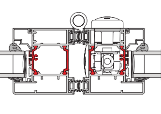
Interlock
