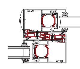
Interlock
