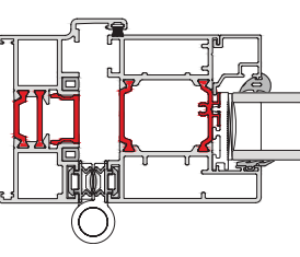
Jam B
